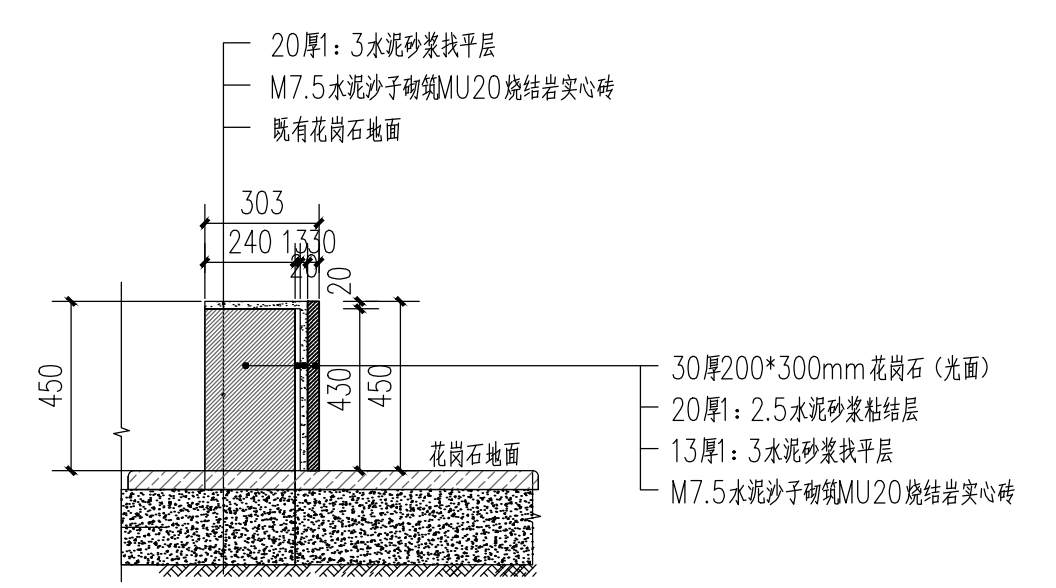
砖砌基础(一) 大样图
