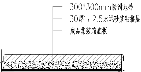
地面做法（一）
