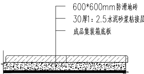
地面做法（二）
