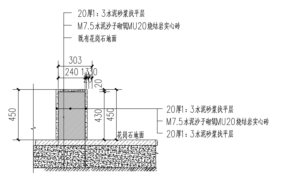
砖砌基础(二) 大样图
