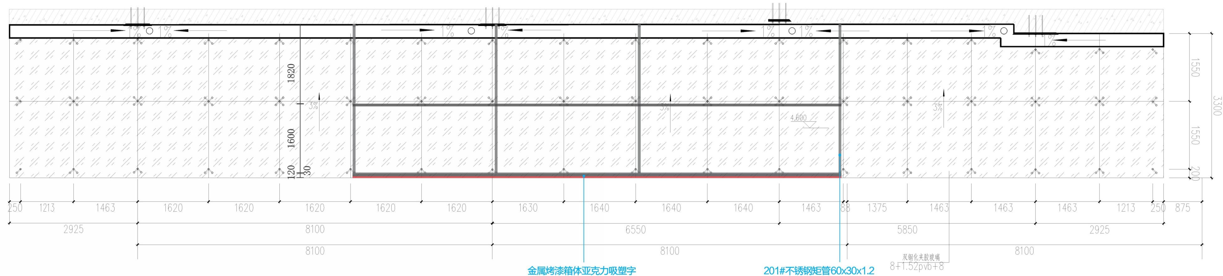
综合楼2号入口吸塑字及辅助钢结构平面图
