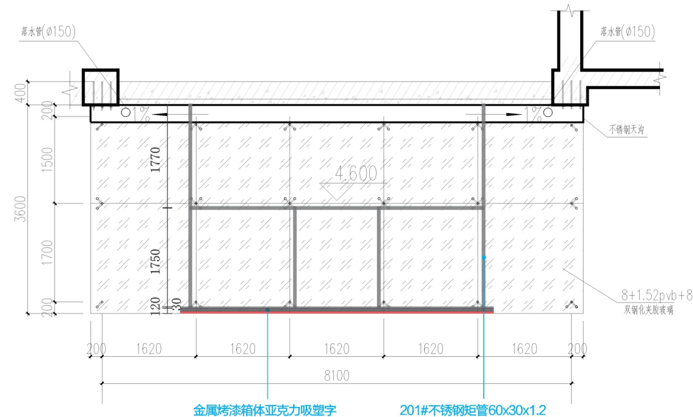
综合楼3号入口吸塑字及辅助钢结构平面图
