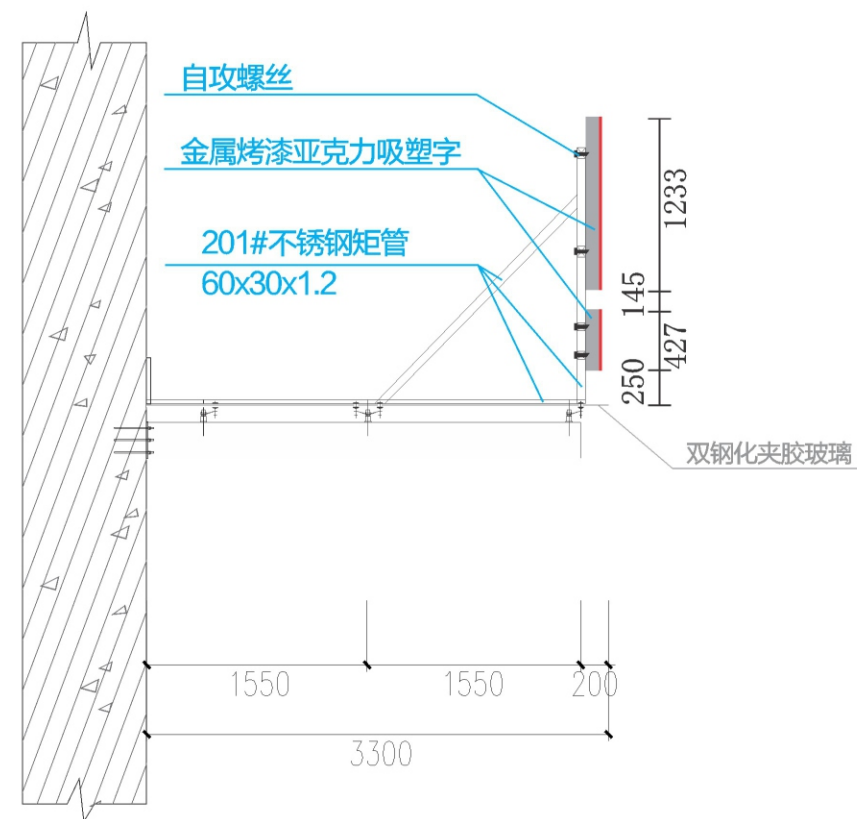
综合楼3号入口吸塑字及辅助钢结构侧面图
