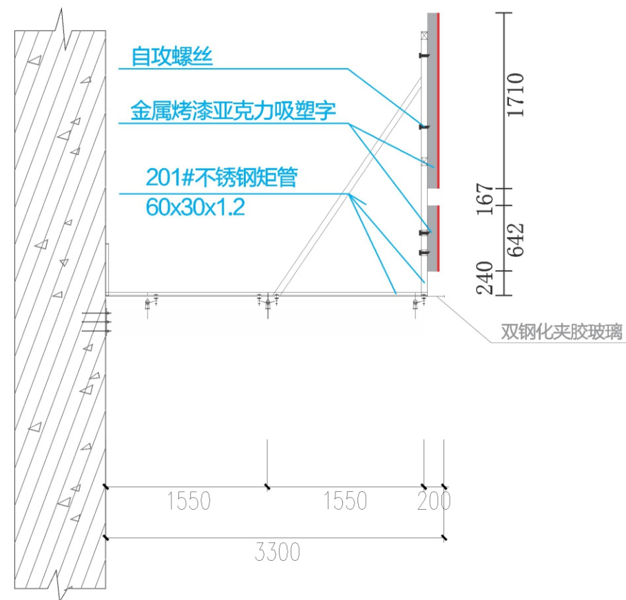
综合楼2号入口吸塑字及辅助钢结构侧面图
