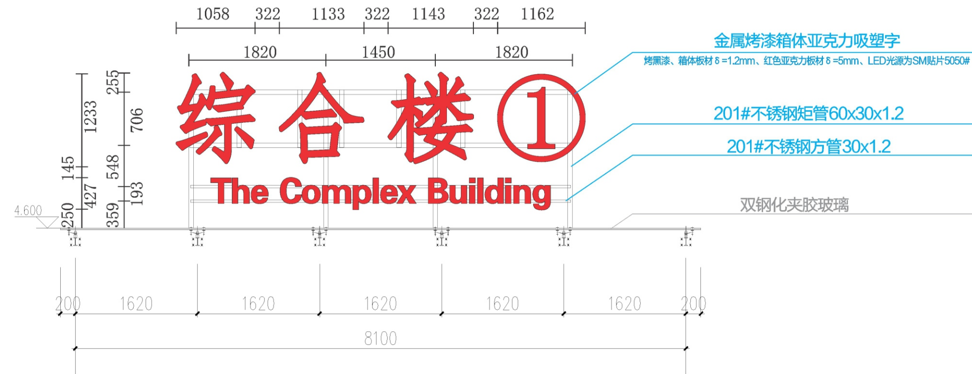
综合楼3号入口吸塑字雨棚正立面安装图
